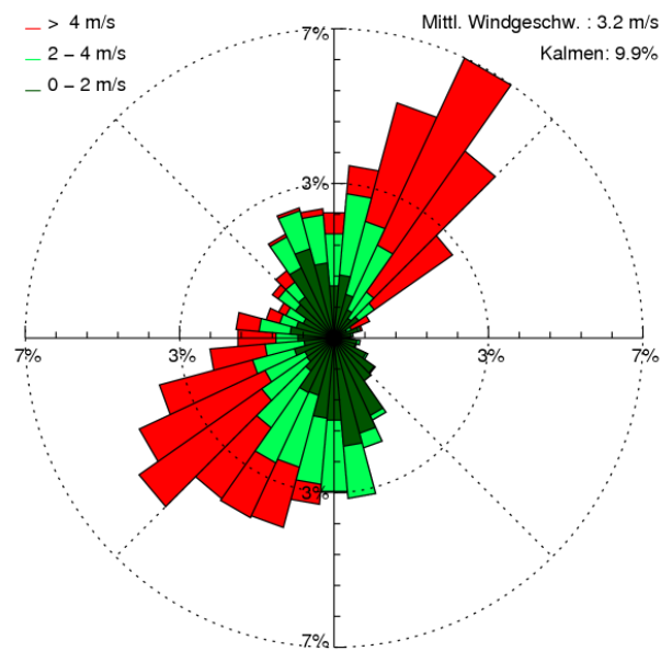
Abbildung 4-5: Windrose für den Standort Eichholz auf 633 m.ü.M.
