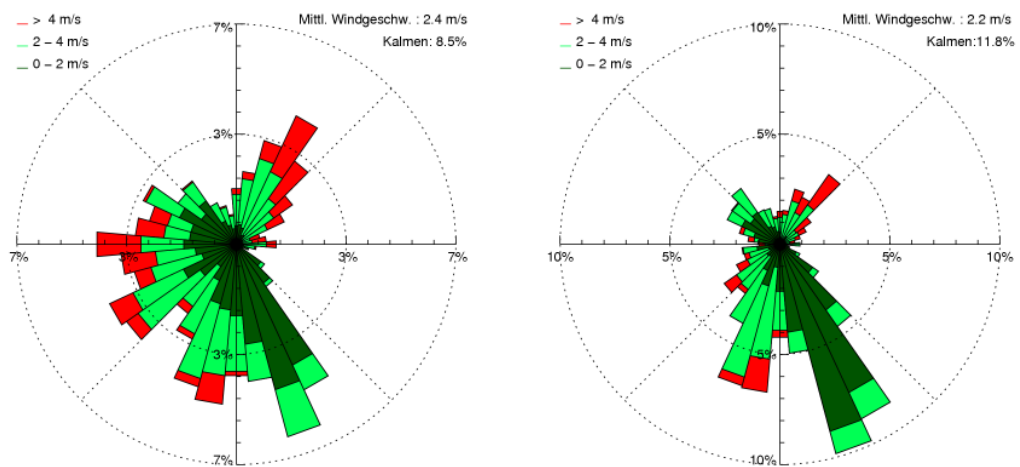
Abbildung 4-4: Windrose für den Standort Filderren auf 573 m.ü.M. für die Perioden von 07 Uhr bis 19 Uhr, Tag (links) und 19 Uhr bis 07 Uhr, Nacht (rechts).
