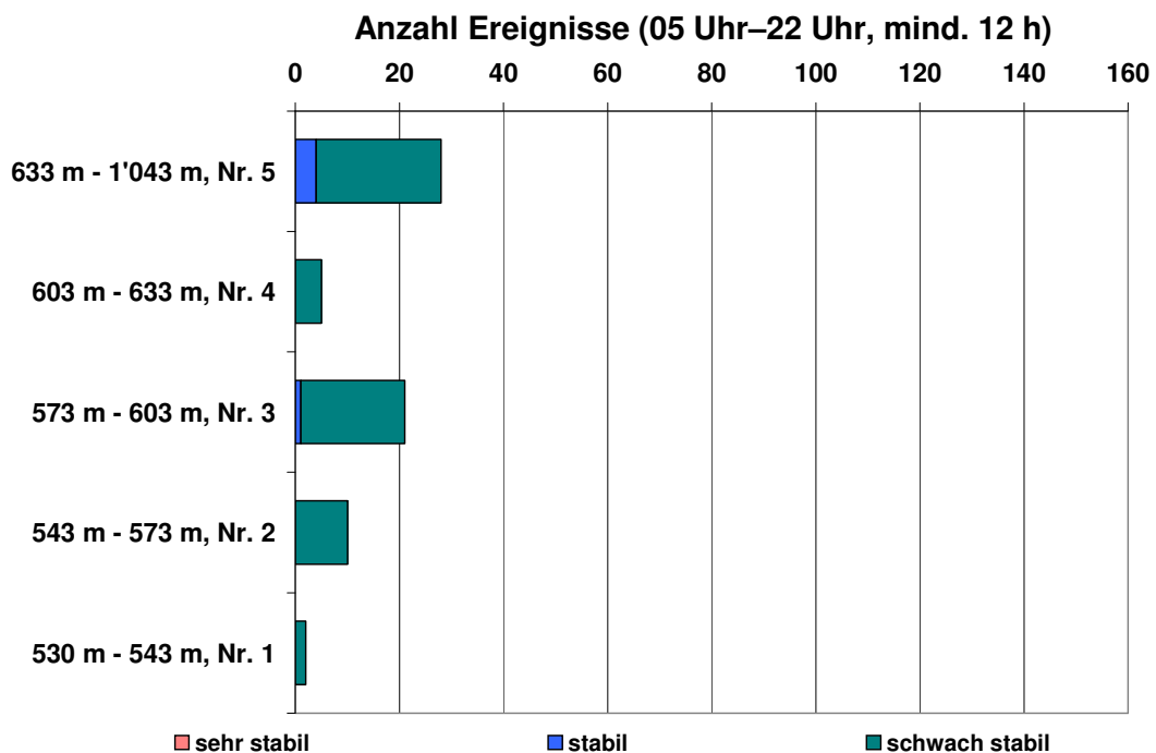
Abbildung 5-9: Graphisch Darstellung der Anzahl Ereignisse pro Luftschicht mit mindestens 12 Stunden dauernder Stabilität während der gesamten analysierten Messperiode für drei Stabilitätskriterien (sehr stabil: rot; stabil: blau; schwach stabil: grün). Für diese Auswertung wurde nur das Zeitfenster 05 bis 22 Uhr berücksichtigt.
